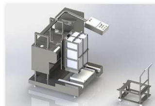
细胞工厂全自动控制机械系统- 两工位机型
