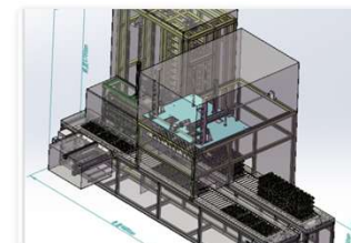
全自动理蛋/胚系统
