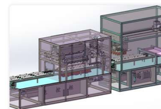
全自动检蛋/胚系统
